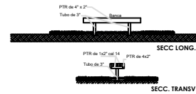
SECC. TRANSV.
