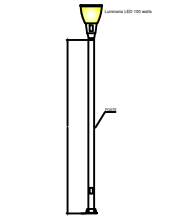
DETALLE DE POSTE 6.00 M. DE ALTURA
