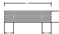
DETALLE DE BANCA
