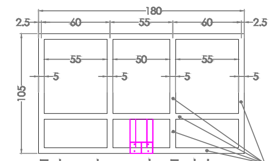
Estructura de Tablero Sin escala - cotas cm.
