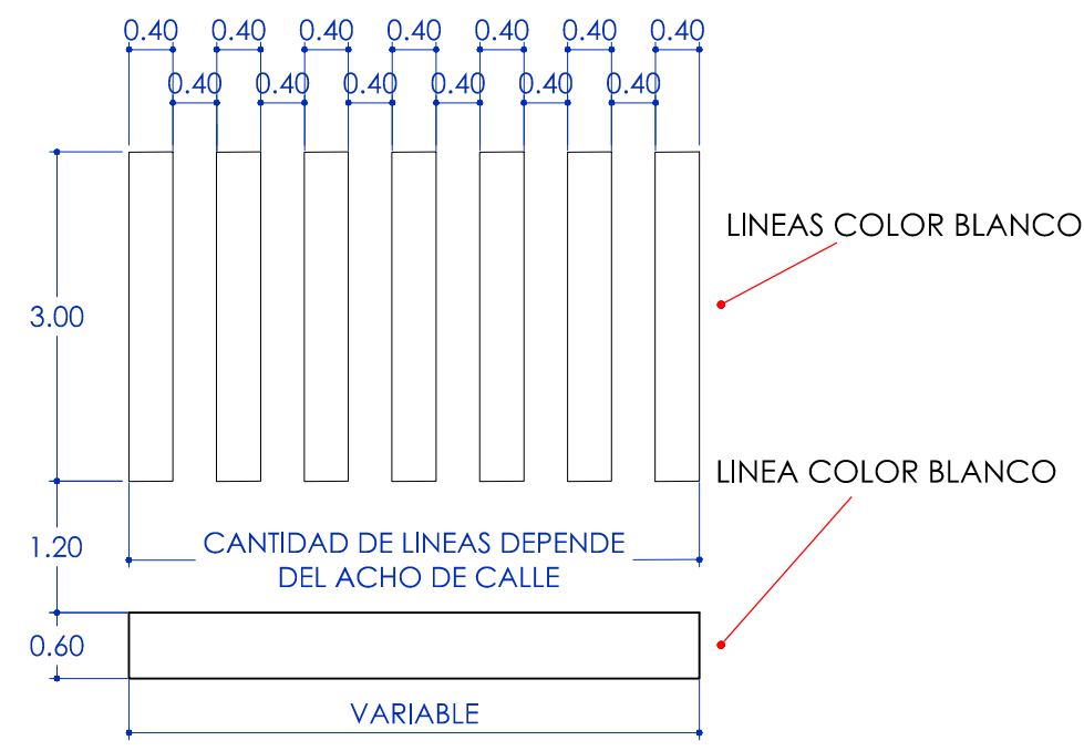
DETALLE PINTURA ZONA PEATONAL SIN ESCALA
