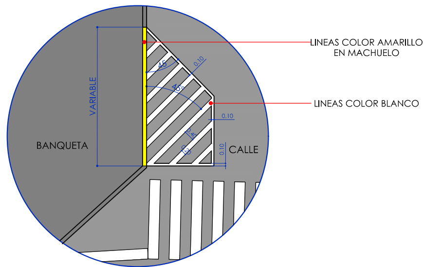
DETALLE PINTURA LINEA DIVISORIA CARRIL SIN ESCALA
